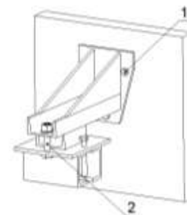
Рисунок 6.1.2- Монтаж консольного кронштейна vрго DL AV02
